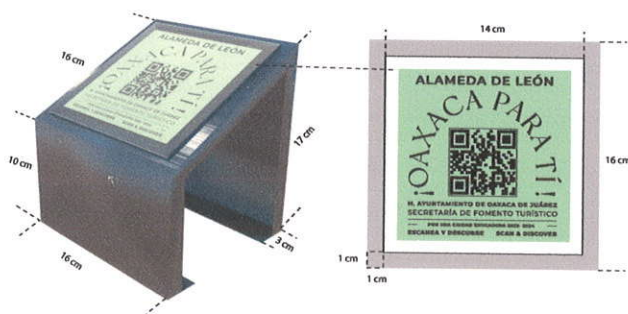
MEDIDAS DE LA BASE Y PLACA
